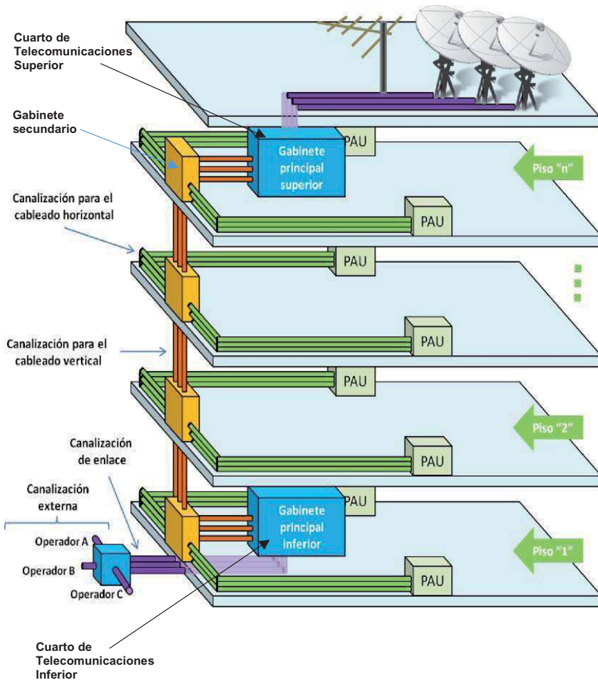
Esquema referencial de canalización de una edificación
